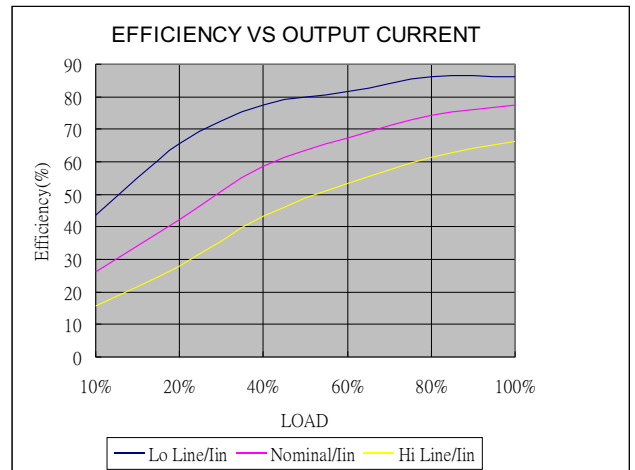
SRBW-4815SD2
